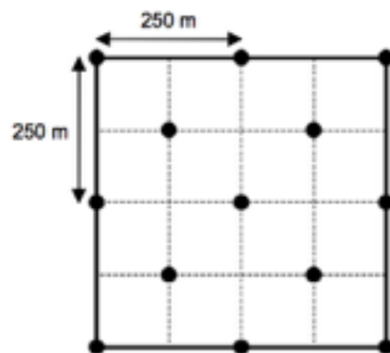
● = Torre de una central de energía eólica Nota: El dibujo no está a escala.
